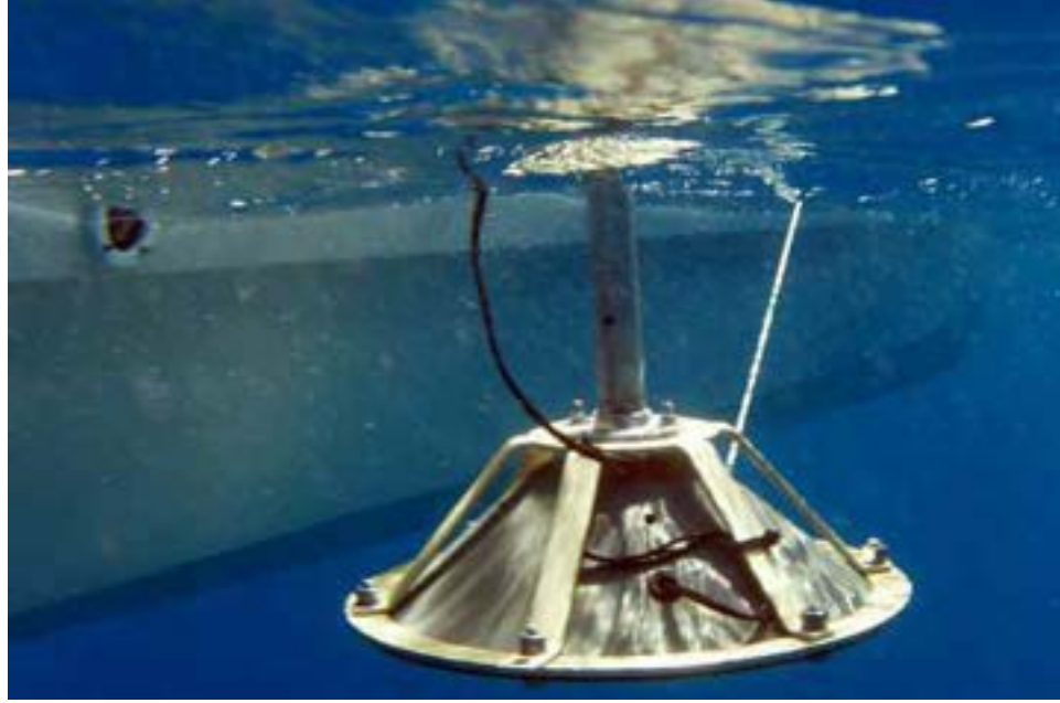
تثبيت محول ذا تردد 10 كيلوهرتز لمسح الطبقات القاعية
